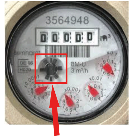
Der Anlaufstern gibt Aufschluss, ob ein Leitungsnetz dicht ist
